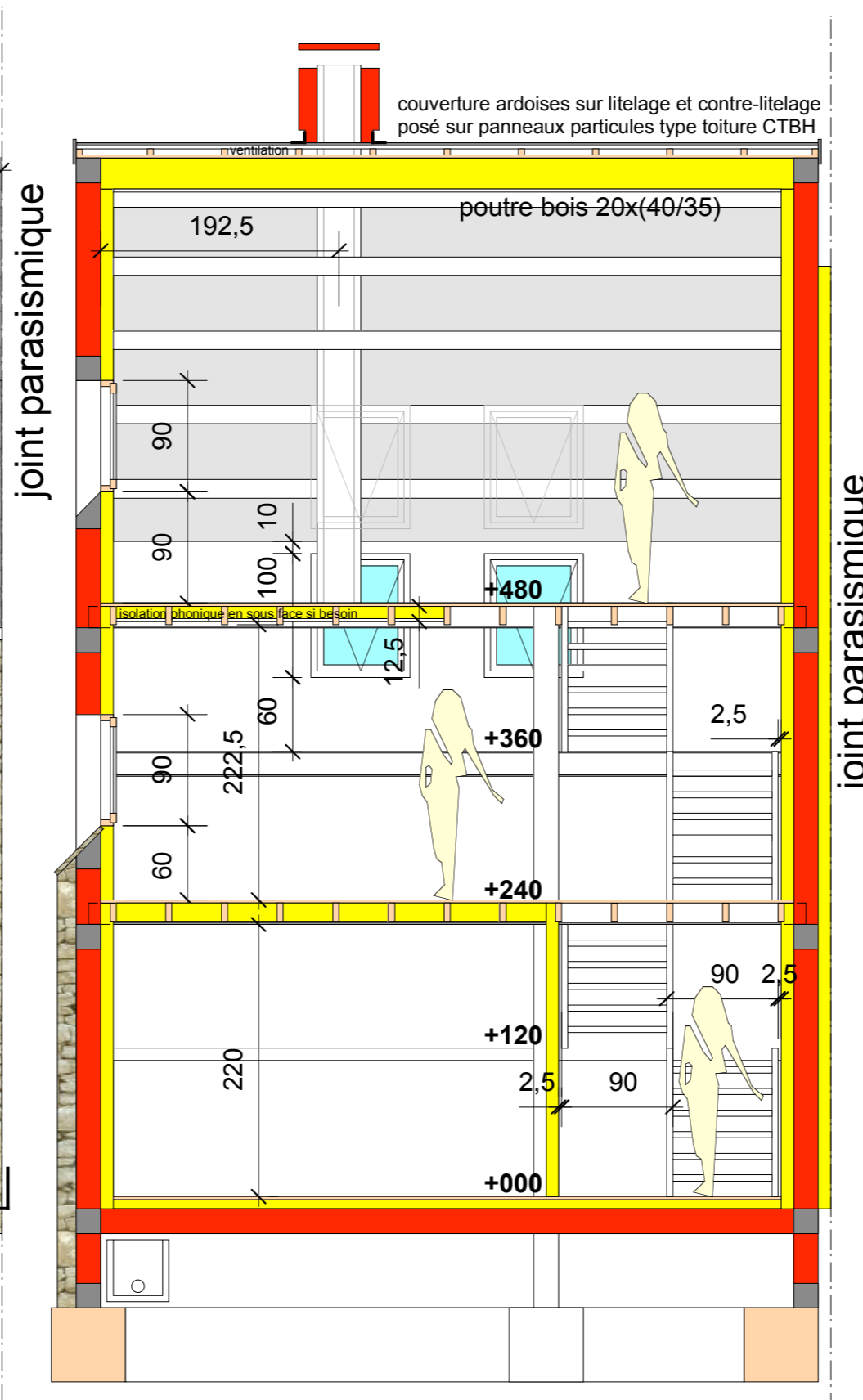
coupe transv.
