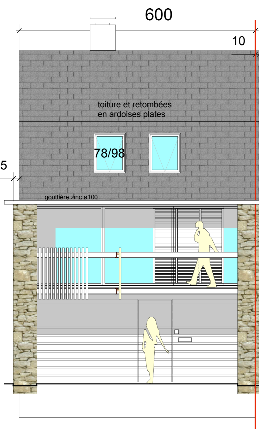
élévation sud
