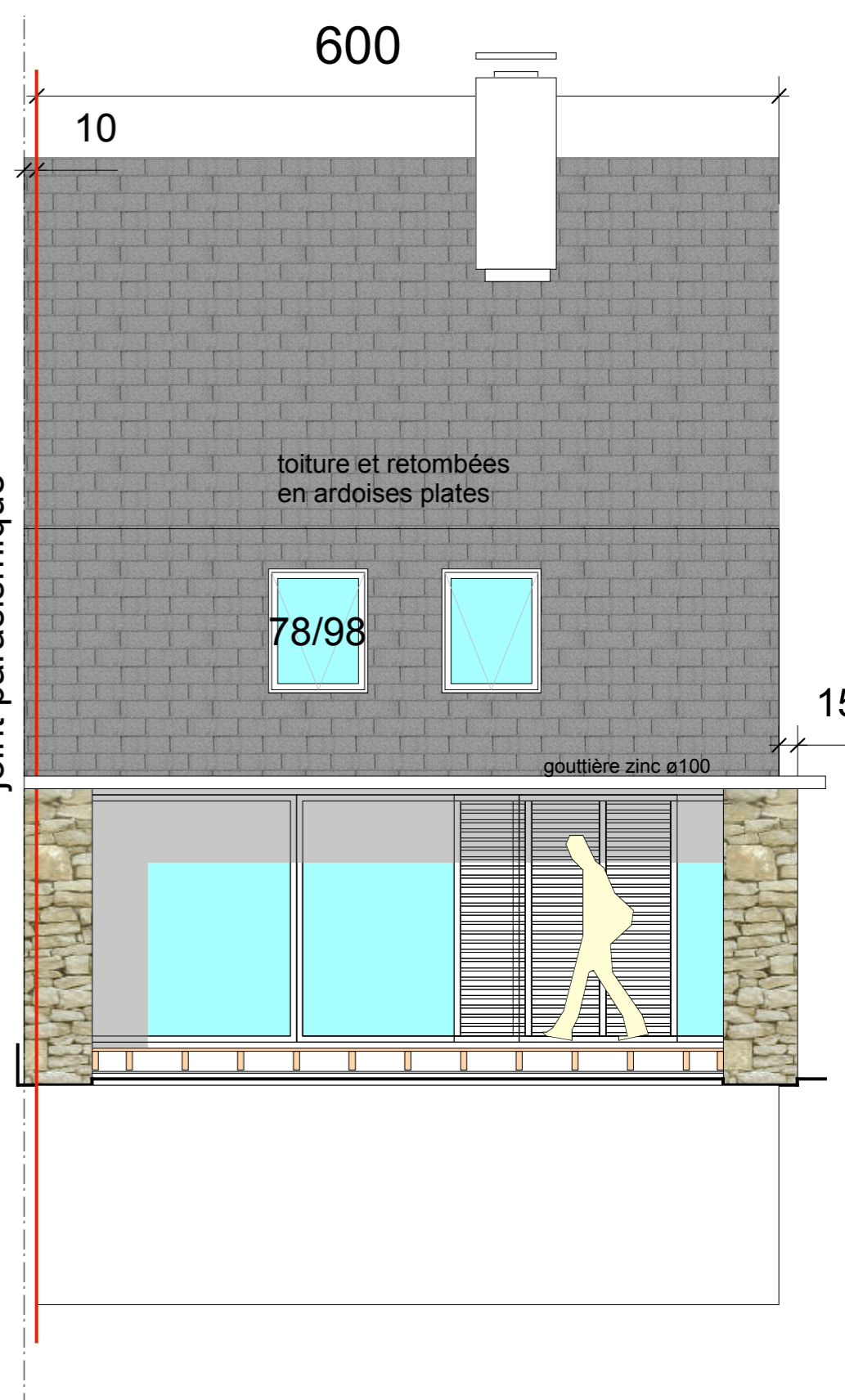
élévation nord
